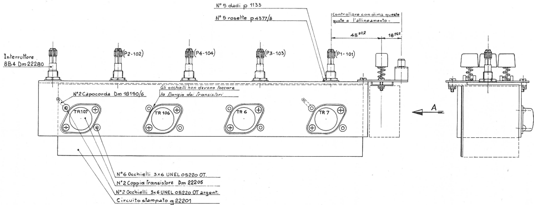
Amplificatore completo
